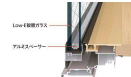
※一般複層ガラス3+A16+3とLow-E複層ガラス6.8+A12+3を比較
